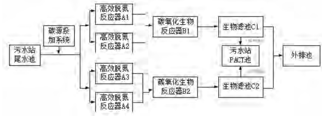
图4.3.2-2 脱氮系统工艺流程图
