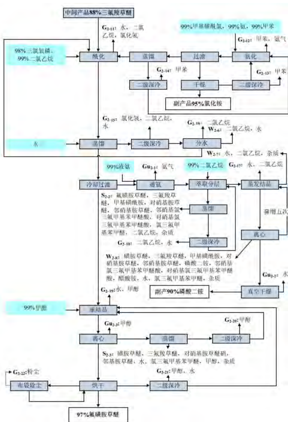
图 4.3-6 氟磺胺草醚、三氟羧草醚工艺流程及产污环节图
