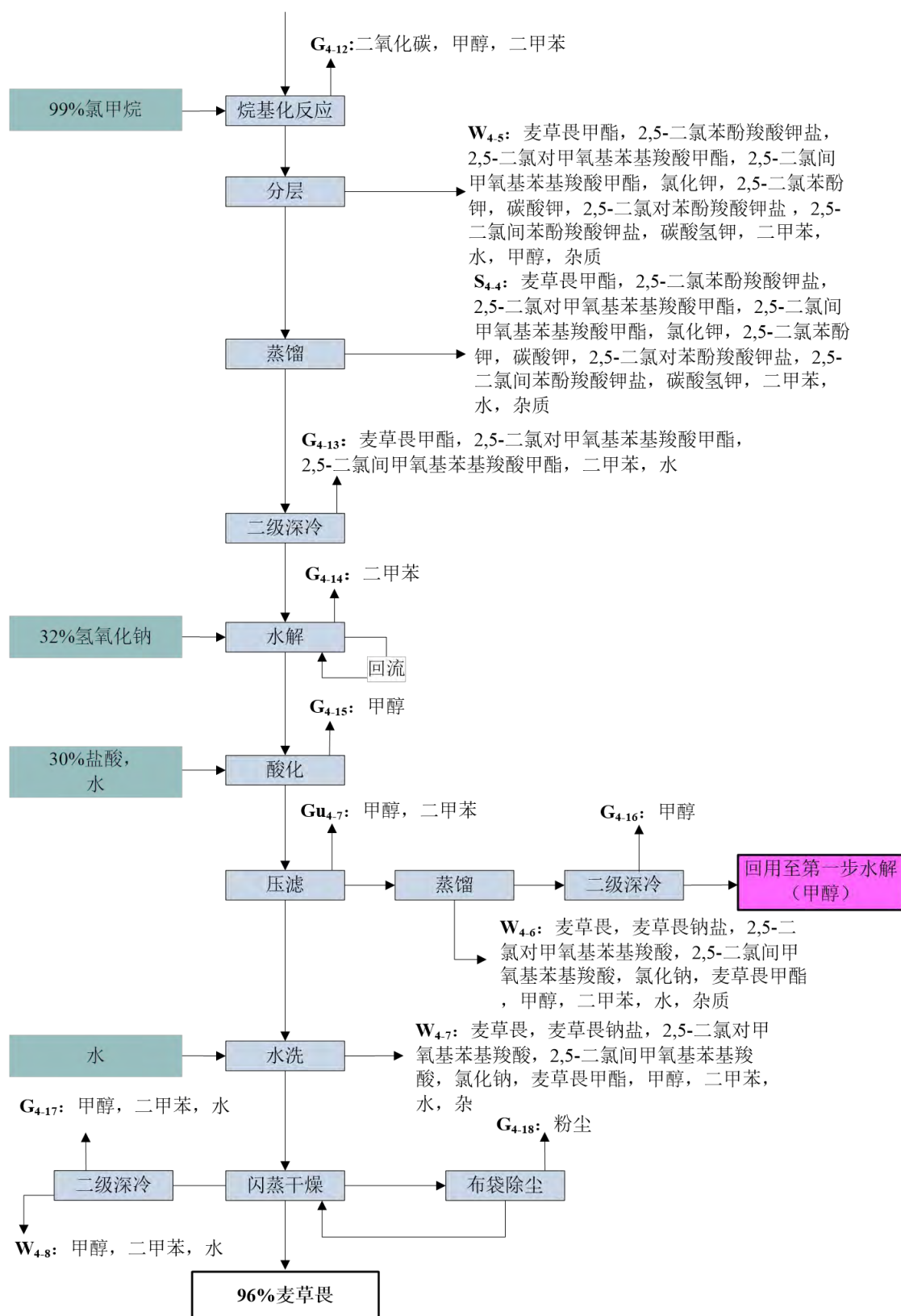
图 4.3-11 麦草畏生产工艺流程图
